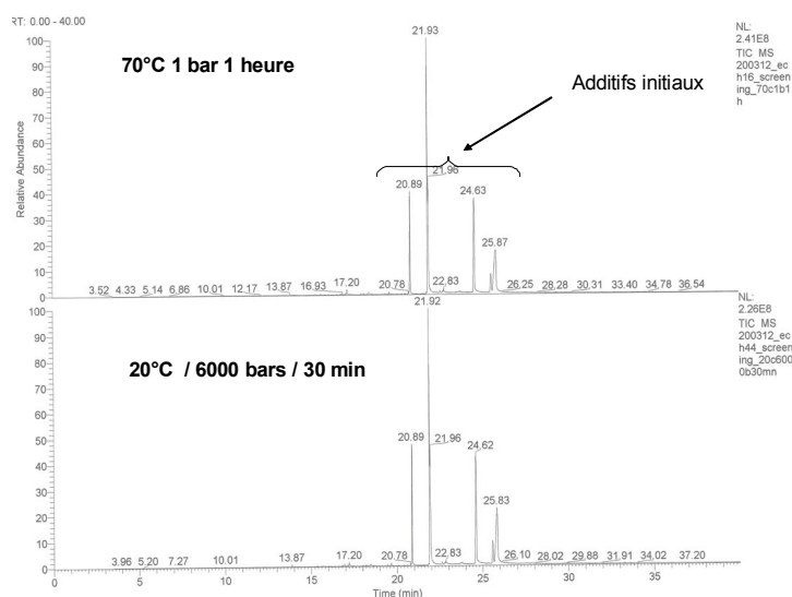
Figure 1 : Concentrations résiduelles des additifs fonctionnels dans le polymère après pasteurisation en autoclave versus PAHP, en présence du simulant huile d'olive
