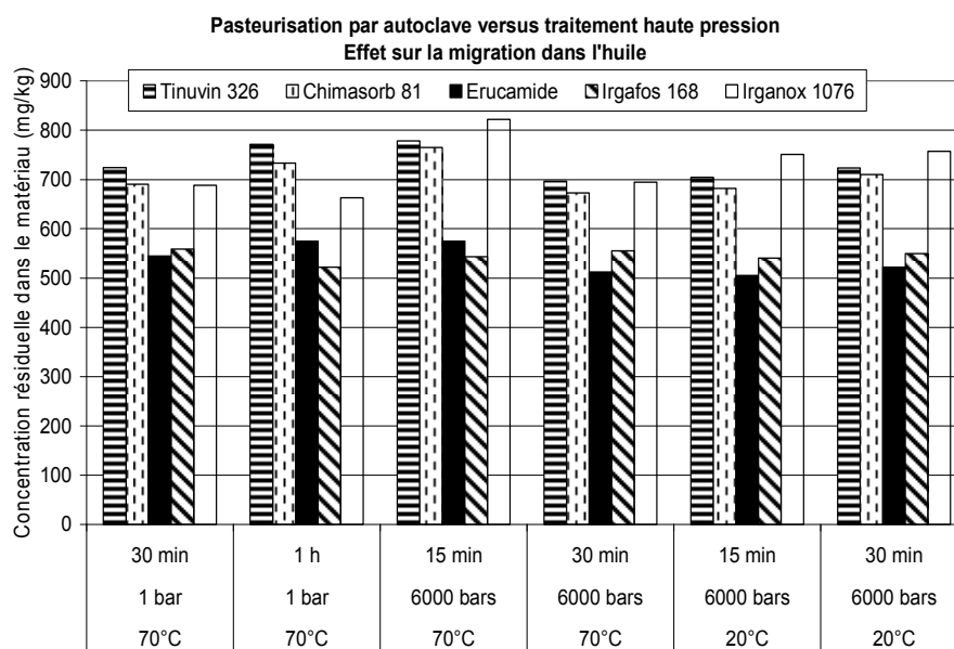
Figure 1 : Concentrations résiduelles des additifs fonctionnels dans le polymère après pasteurisation en autoclave versus PAHP, en présence du simulant huile d'olive
