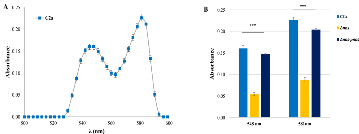
Figure 1 : Evaluation de la production de monoxyde d'azote (NO) via la formation de nitrosomyoglobine. A) Spectre d'absorbance obtenu après conversion de metmyoglobine en nitrosomyoglobine pour la souche C2a, montrant deux pics d'absorption à 548nm et 581nm. B) Mesure de l'absorbance à 548 nm et 581 nm pour la souche C2a, le mutant \Delta nos et le mutant complétement \Delta nospRBnos . ***, p < 0.001 .
